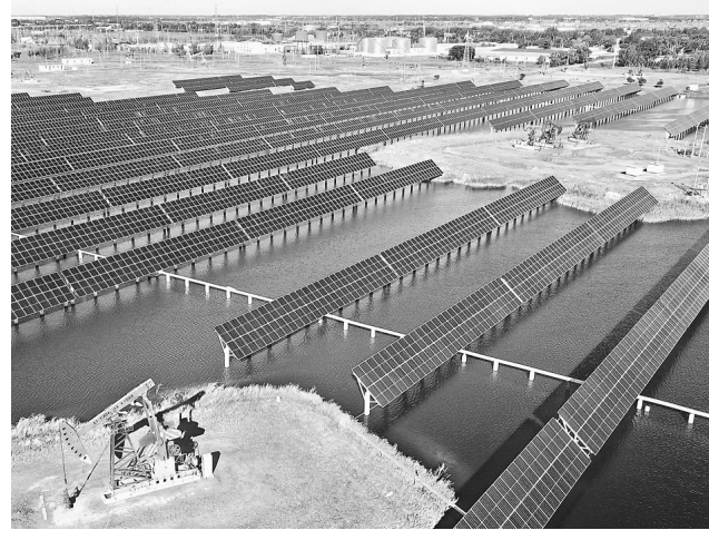
这是9月19日拍摄的大庆油田星火水面光伏电站局部(无人机照片)。
